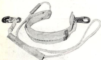
ST#522 ロープ式命づな
