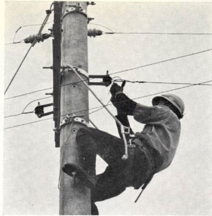
昇柱用安全バンドの使用状態 ST#508型 ST#509型
