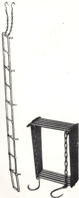
鋼製はしご折畳式
