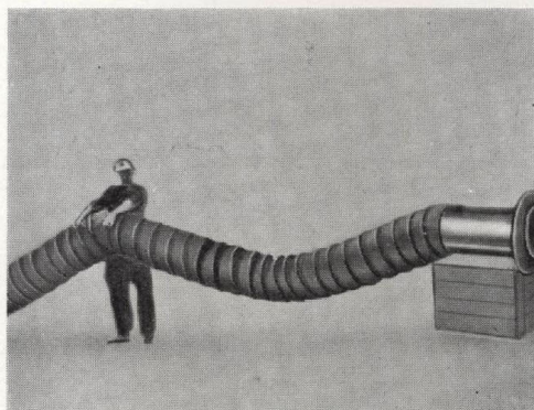
螺旋式風管でタンクやマンホールからガスを吸引する方法
