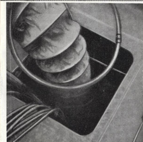
造船所において船体建造中マンホールよりガス気を外部に排出中の写真です。
