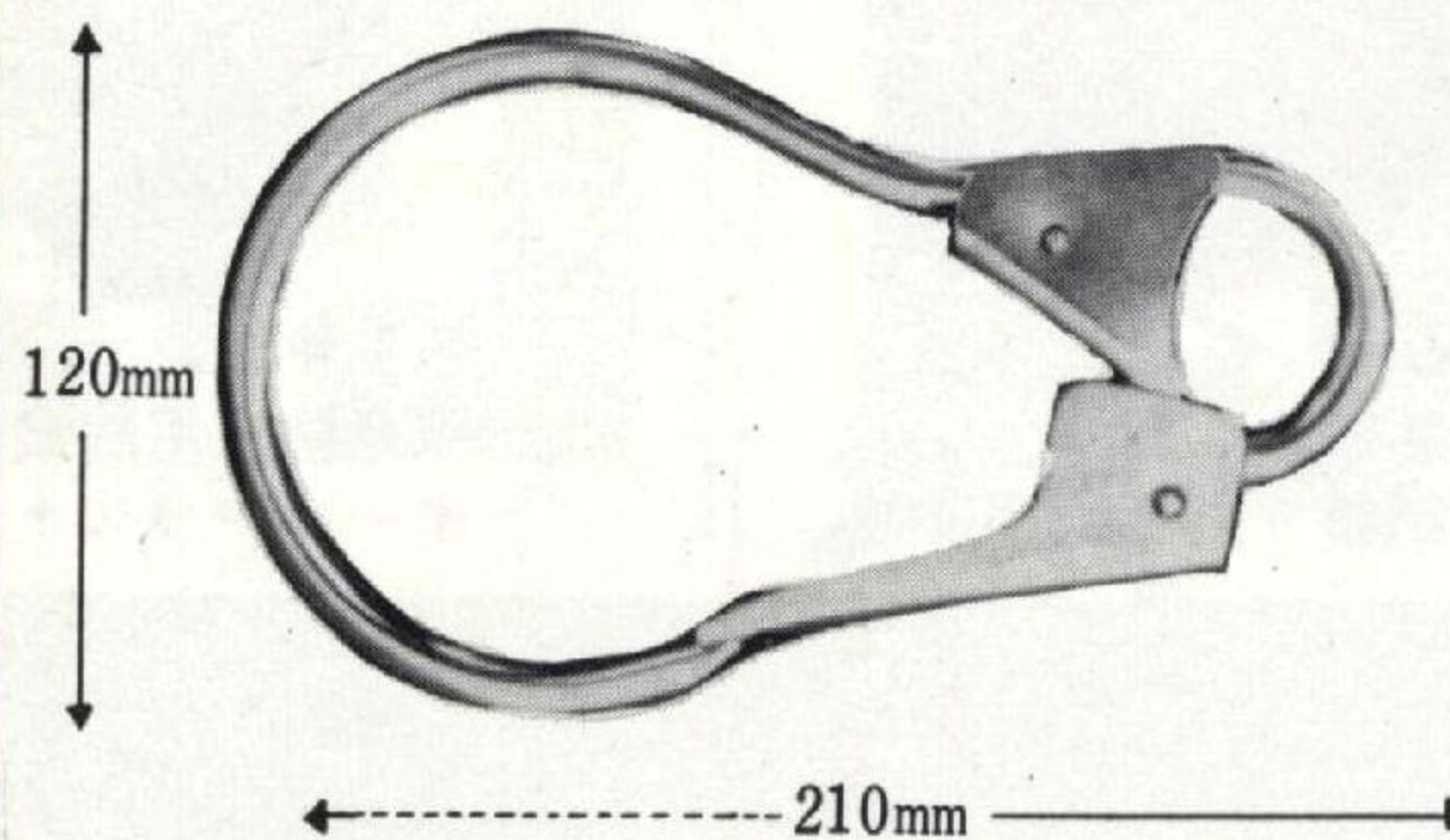
鉄筋作業用大フック
