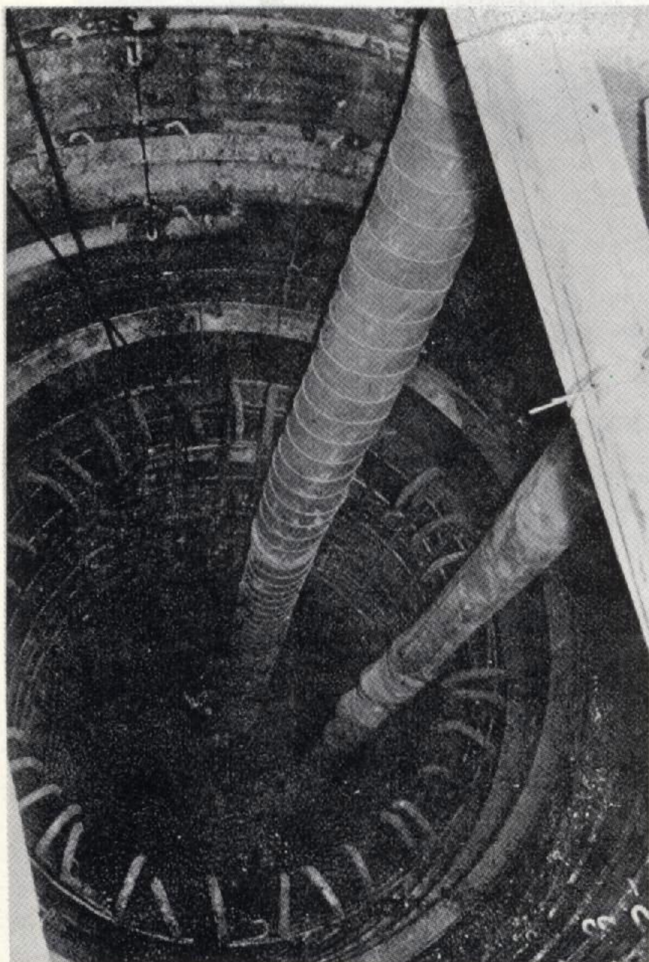
深礎工法に於ける送風状況
