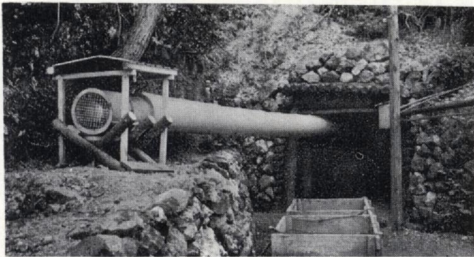
鉱道内送風実況
