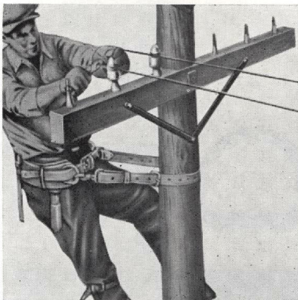
安全バンドを着帯して作業中の写真です。
