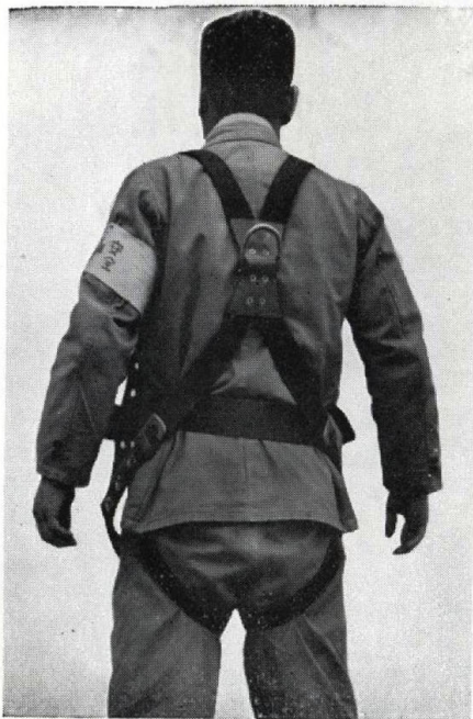
タニサワ式 # 512 肩と股懸付安全吊帯 (ビニロン製)
