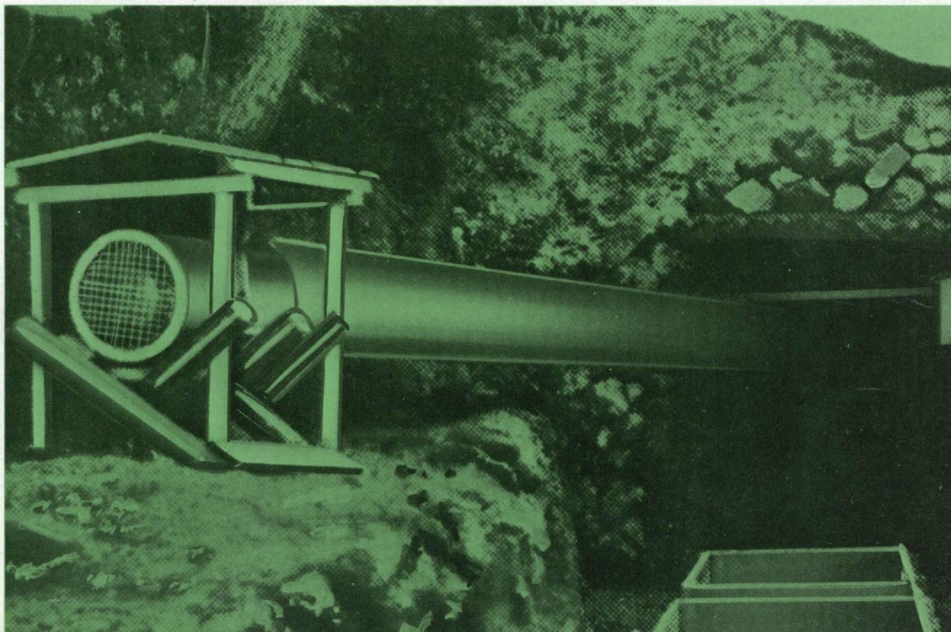
▼ 鉱山で使用中のタニザワ式ナイロン布風管と小型電動送風機の実況
