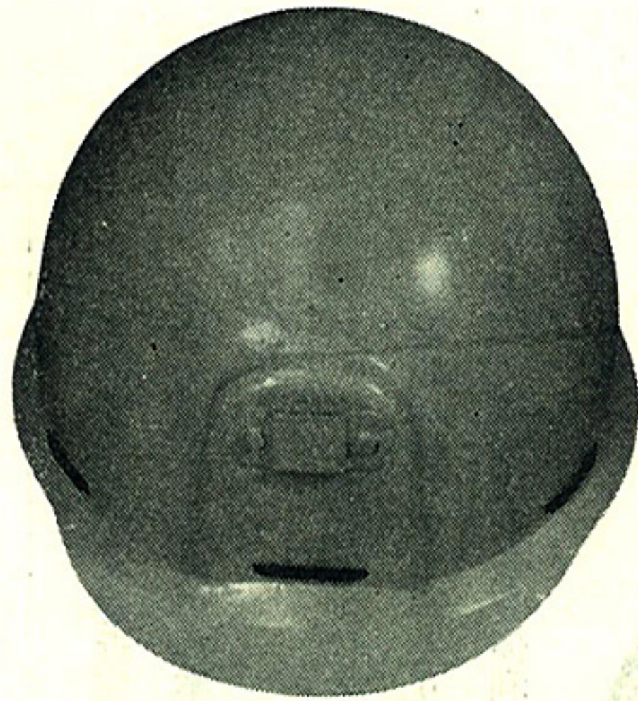
布積層ベークライト製保安帽 ゴムクッション式内装付 ST # 122 定価 ¥ 650.
