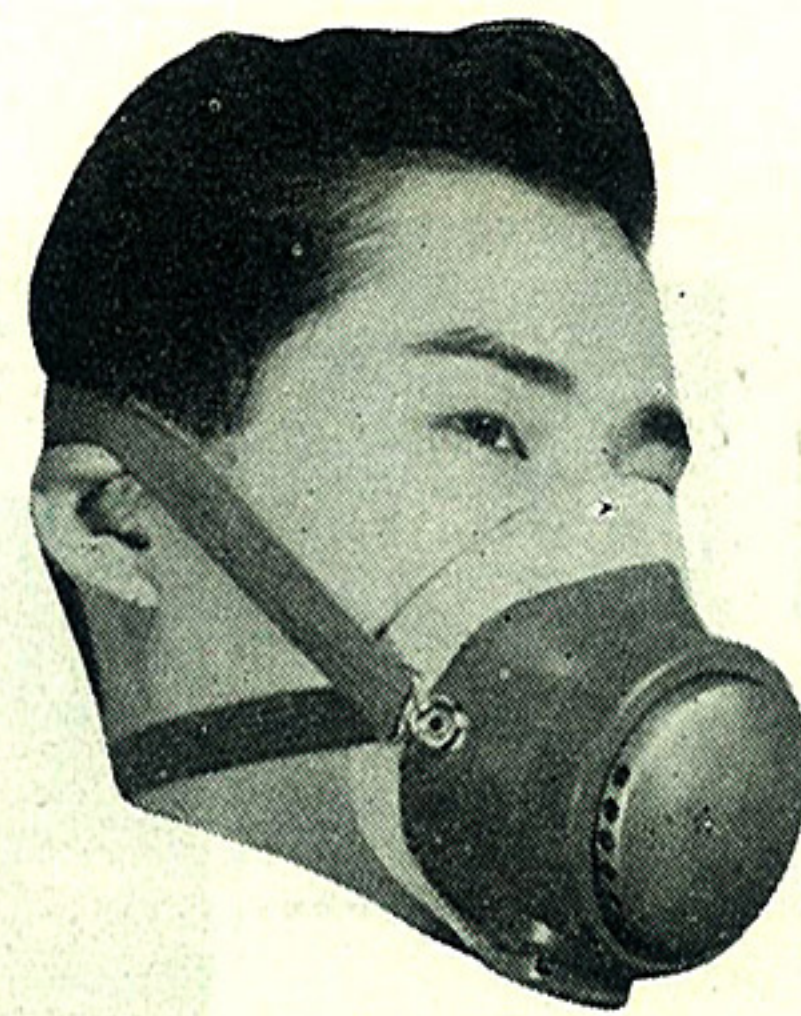
防じんマスク S T # 206-B 定価 ¥ 350. 4種合格品 汚じん効率 73.8% 通気抵抗 4.6 耗
